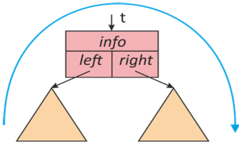
In-order обход
